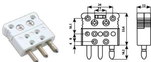
zástrčka , teplotní odolnost do 220 °C standartní velikost , duté vývody
