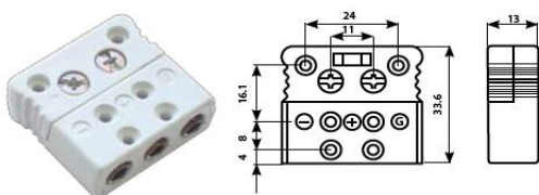
zásuvka , teplotní odolnost do 220 °C standartní velikost
