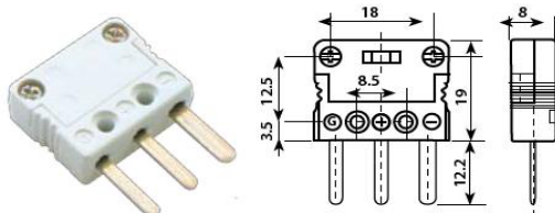
zástrčka , teplotní odolnost do 220 °C velikost mini
