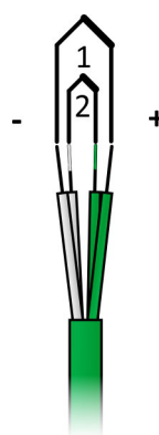
Obrázek 11.8: Zapojení dvojitého termočlánu
