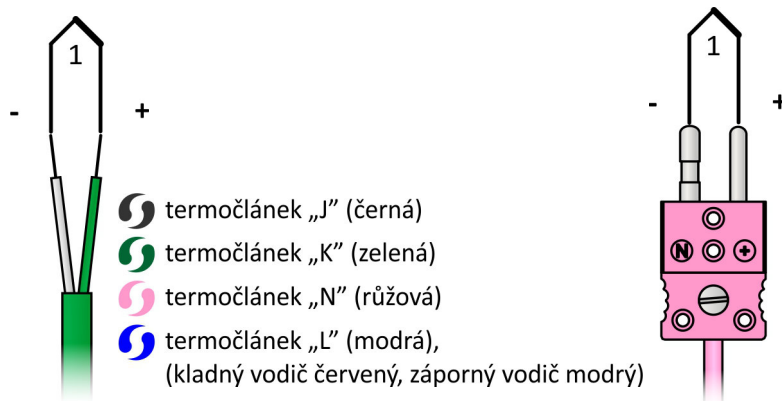
Obrázek 13T.2: Zapojení jednoduchého termočlánku
