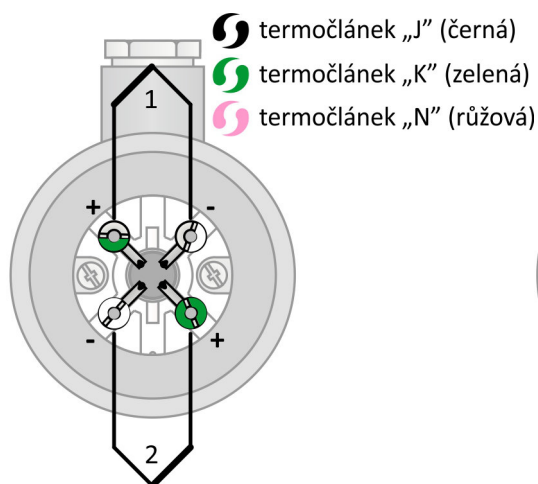
Obrázek 7UC.3: zapojení dvojitého termočláneku
