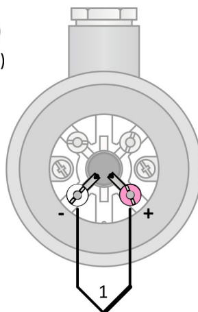
Obrázek 7UC.4: zapojení jednoduchého termočláneku
