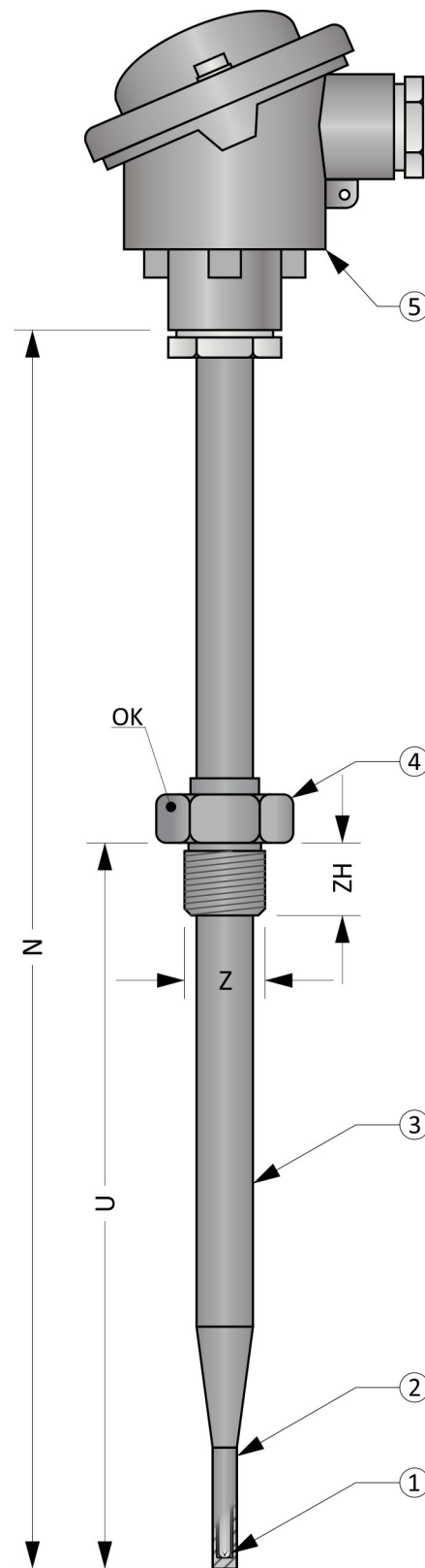
Obrázek 8VR.1: MTC8VR
