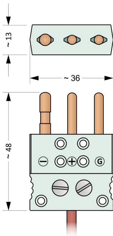
Obrázek 11.6: MTCK-3S
