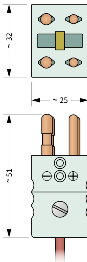
Obrázek 11.7: MTCK-4S
