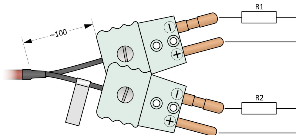
Obrázek 12.19: 2 x RTD v dvouodičovém zapojení se dvěma konektory
