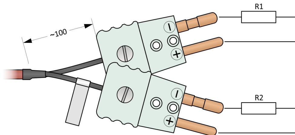
Obrázek 13T.19: 2 x RTD v dvouodičovém zapojení se dvěma konektory
