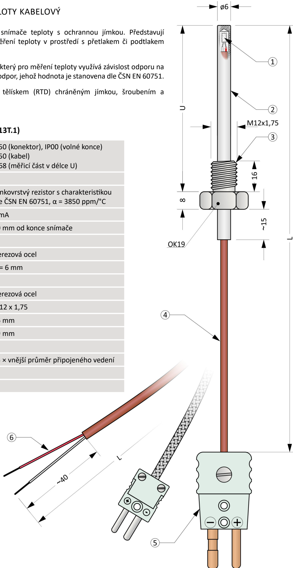
Obrázek 13T.1: MTR13T
