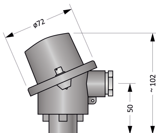
Obrázek 14.3: Hlavice BH
