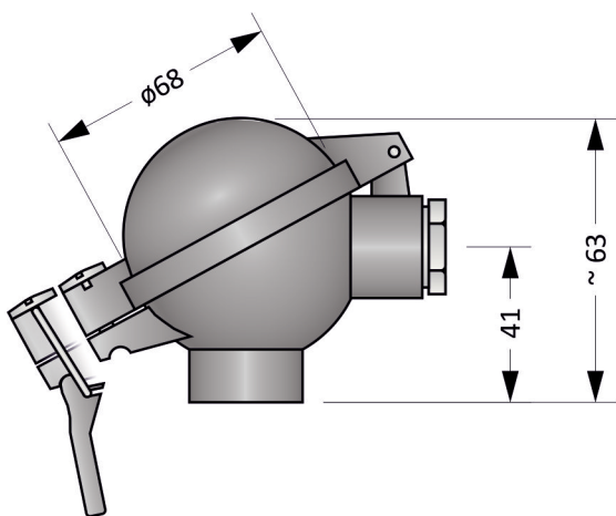
Obrázek 9.4: Hlavice BUZ
